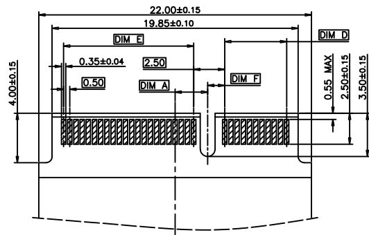
BOTTOM SIDE
