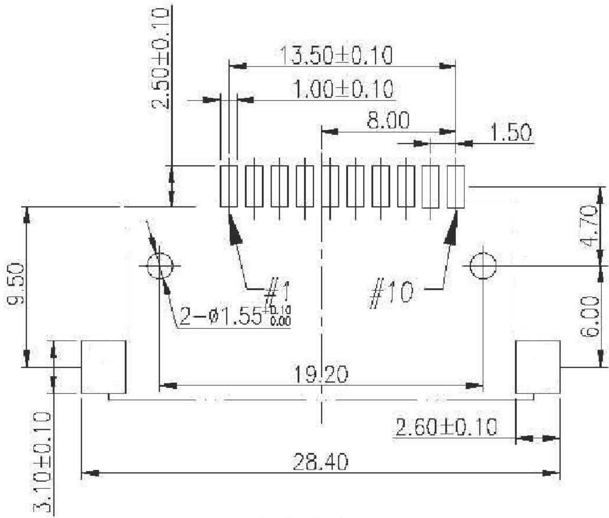
P.C.B Layout
